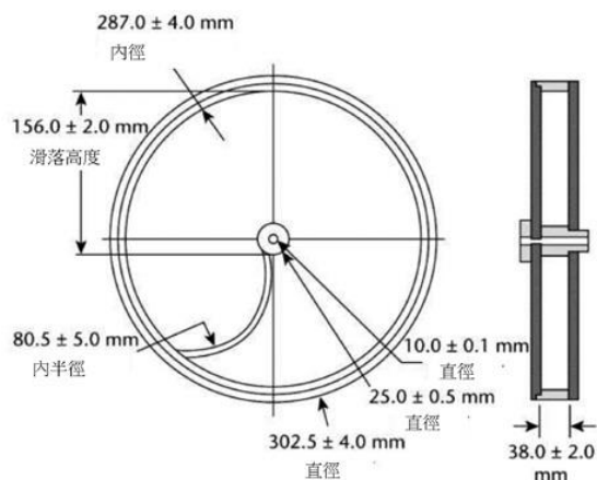
錠劑脆度試驗法裝置圖
