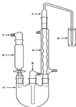
圖二 方法五之裝置
