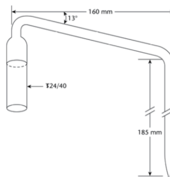
圖三 方法五裝置中之起泡器 F
