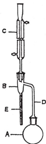
圖一 甲苯蒸餾裝置
